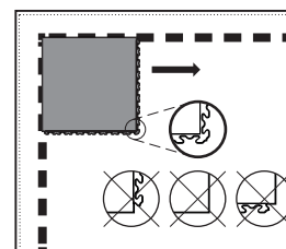
Abb. Nr. 3 Verlegungsrichtung der Fliesen INVISIBLE, BUSINESS
