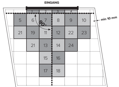
Abb. Nr. 2 Verlegung von Fortelock INVISIBLE, BUSINESS
